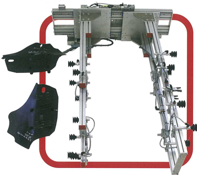
Greifer für 3 Plattenwerkzeug EOAT for Stackmould
