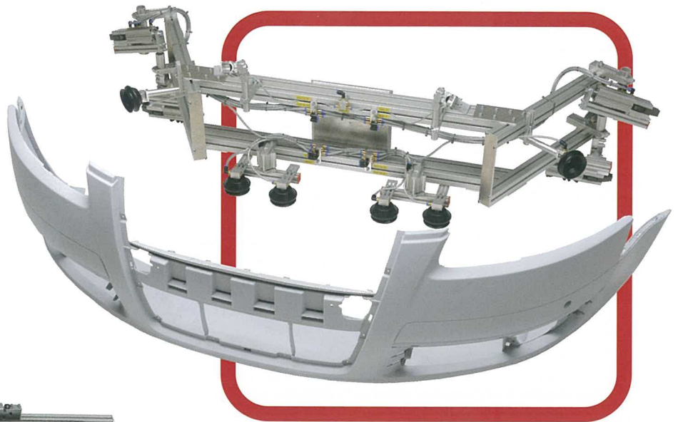
Greifer für Stoßfänger EOAT for Bumper
