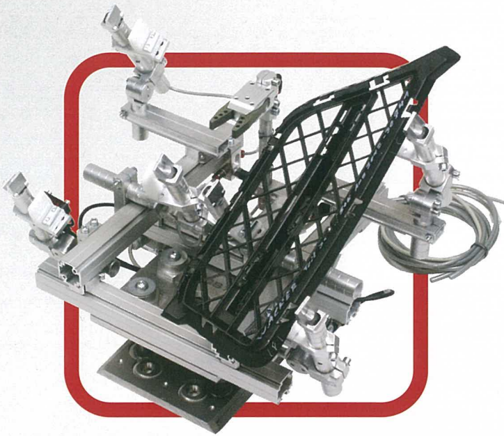
PreciGrip-Greifer für Abdeckung PreciGrip-EOAT for housing
