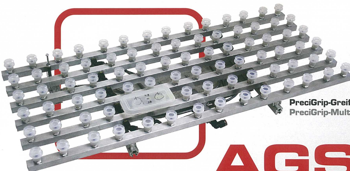
PreciGrip-Greifer für Grill PreciGrip-EOAT for Carpart
